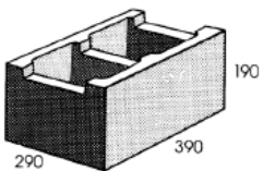
30.42 Top groove
